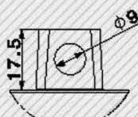
Detail A Scale: 4:5 UT type
