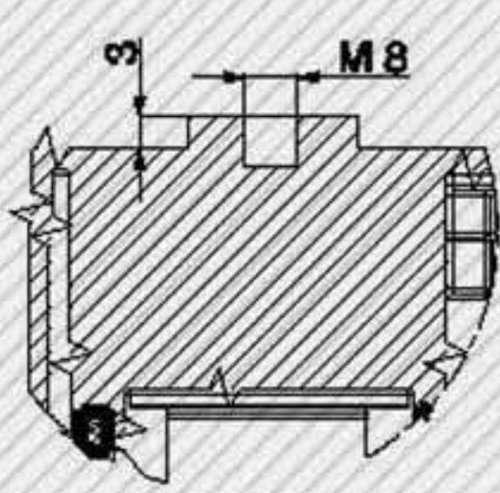
Detail A Scale: 1:1 Insert type
